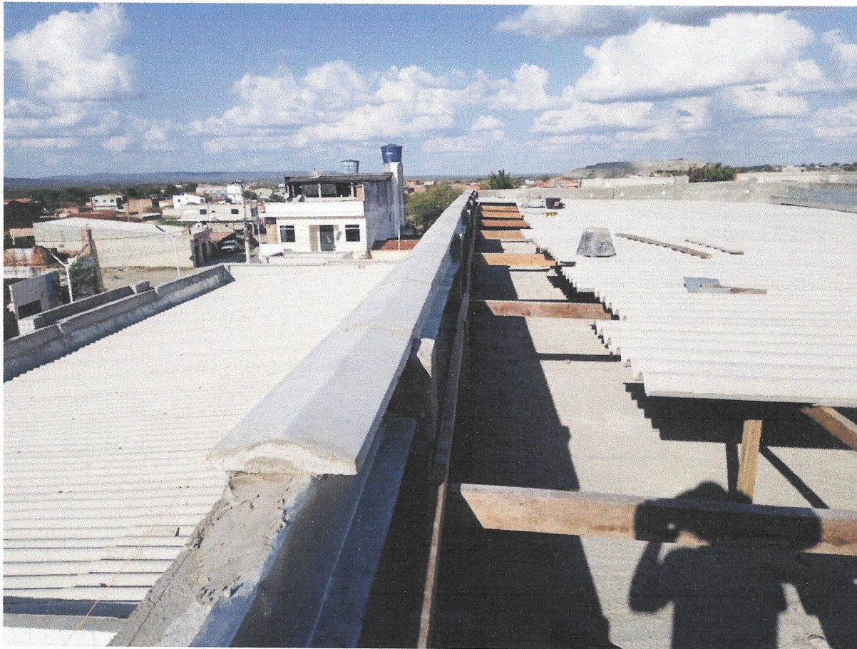
FOTO 12 - CHAPIM DE CONCRETO PRÉ-MOLDADO
