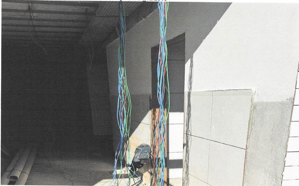
FOTO 46 - ELETRODUTO FLEXÍVEL CORRUGADO, PVC, DN 32 MM (1"), PARA CIRCUITOS TERMINAIS, INSTALADO EM PAREDE - FORNECIMENTO E INSTALAÇÃO. AF_12/2015
