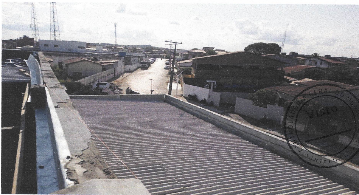
FOTO 12 - CHAPIM DE CONCRETO PRÉ-MOLDADO
